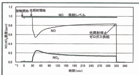
光触媒材料の空気浄化性能試験結果報告書（窒素酸化物の除去性能） 試験機関：一般社団法人 関西環境管理技術センター
